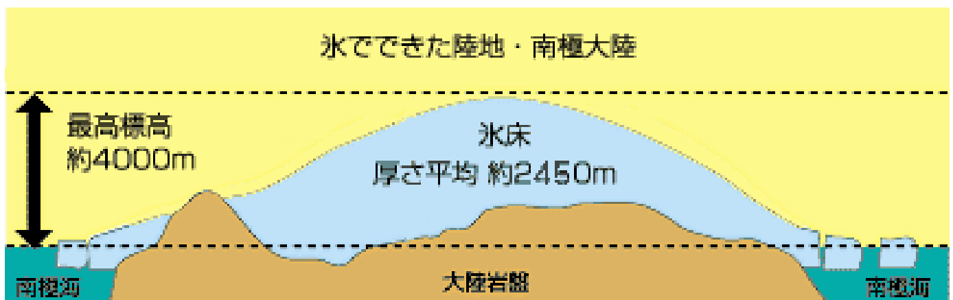
南極大陸の断面図（環境省のHPより）
